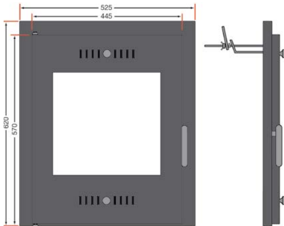
Porto Stove Door Dimensions
